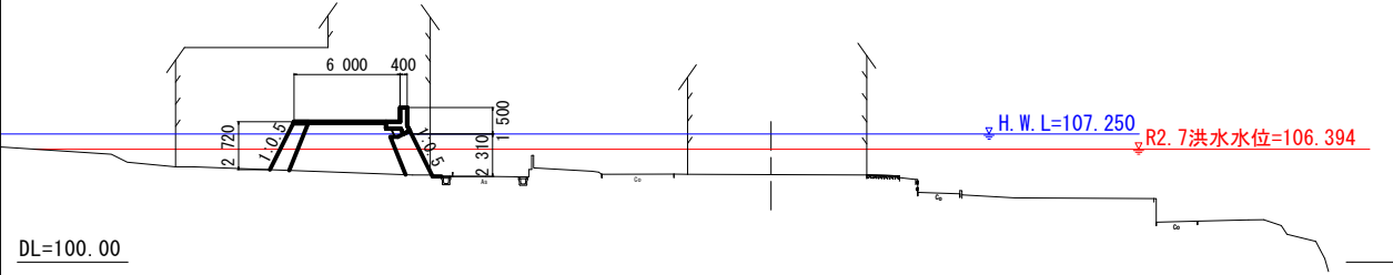
代表断面 (A-A断面)
