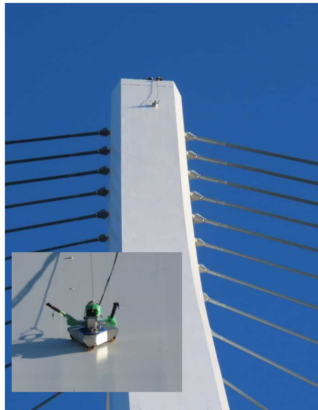
▲マグネット式全方位点検ロボットによる点検状況 (主塔上部側面)
