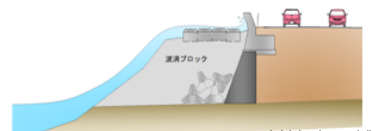
既設消波ブロックが 設置されている箇 所は、“フレキャスト護 岸”構造を採用
