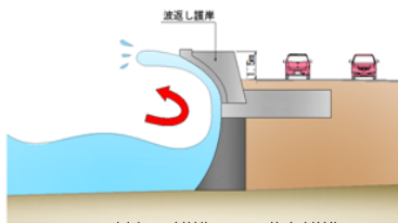
波返し構造：フレア護岸構造 (消波ブロックが設置されていない箇所)
