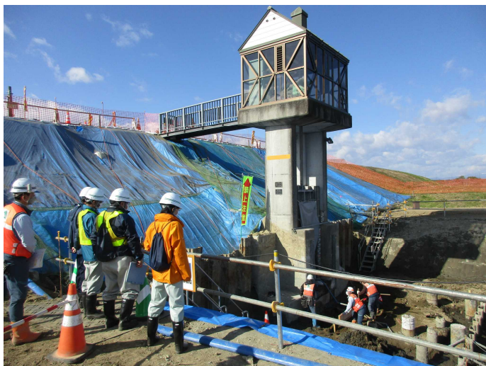
江合川 荒雄排水樋管改修工事現場
