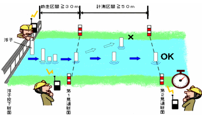
洪水時の流量観測（高水流量観測）
