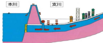
大曲川及び広瀬川排水施設(北上市)で採用
