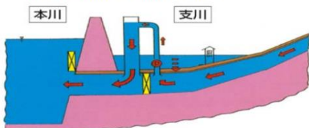
後川排水施設(花巻市)で採用
