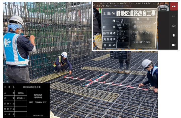
遠隔臨場による鉄筋出来形測定
