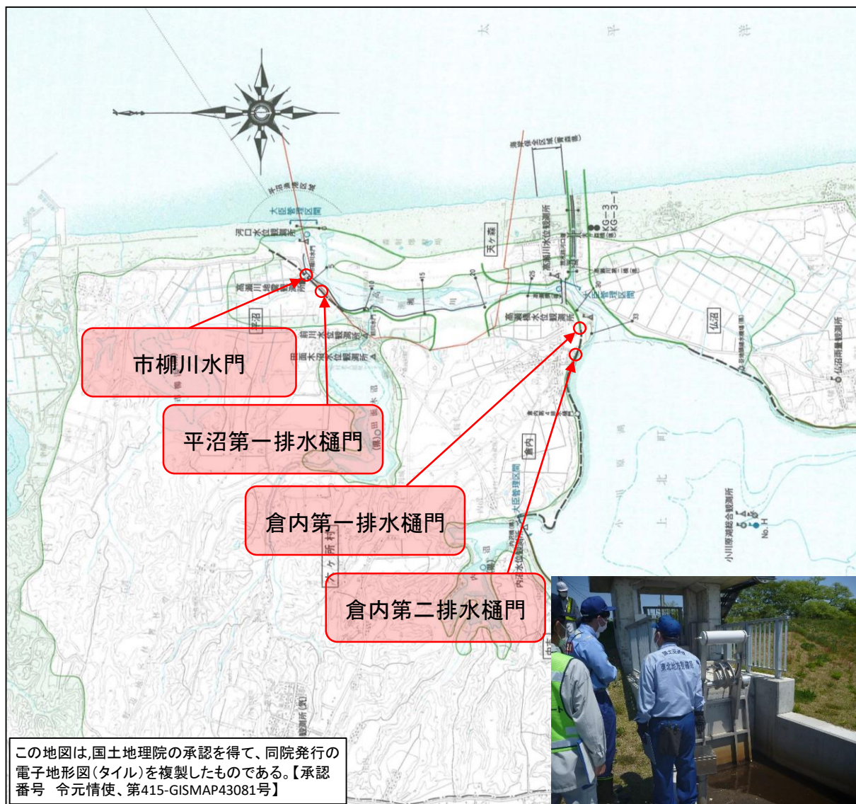
排水樋門の点検状況
