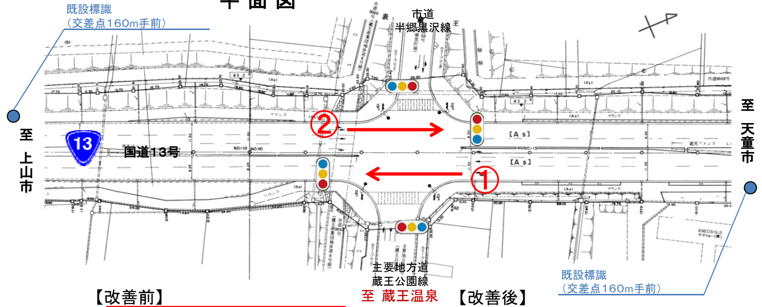
平面図
