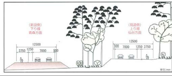
【上下線分離(松並木)区間】
