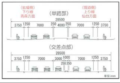
【拡幅区間(菓子市街地部)】
