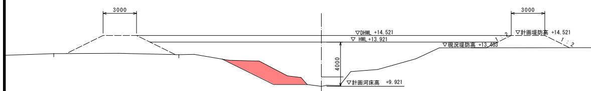
標準断面図A-A
