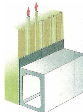
— 型枠支持材撤去概念図 —
