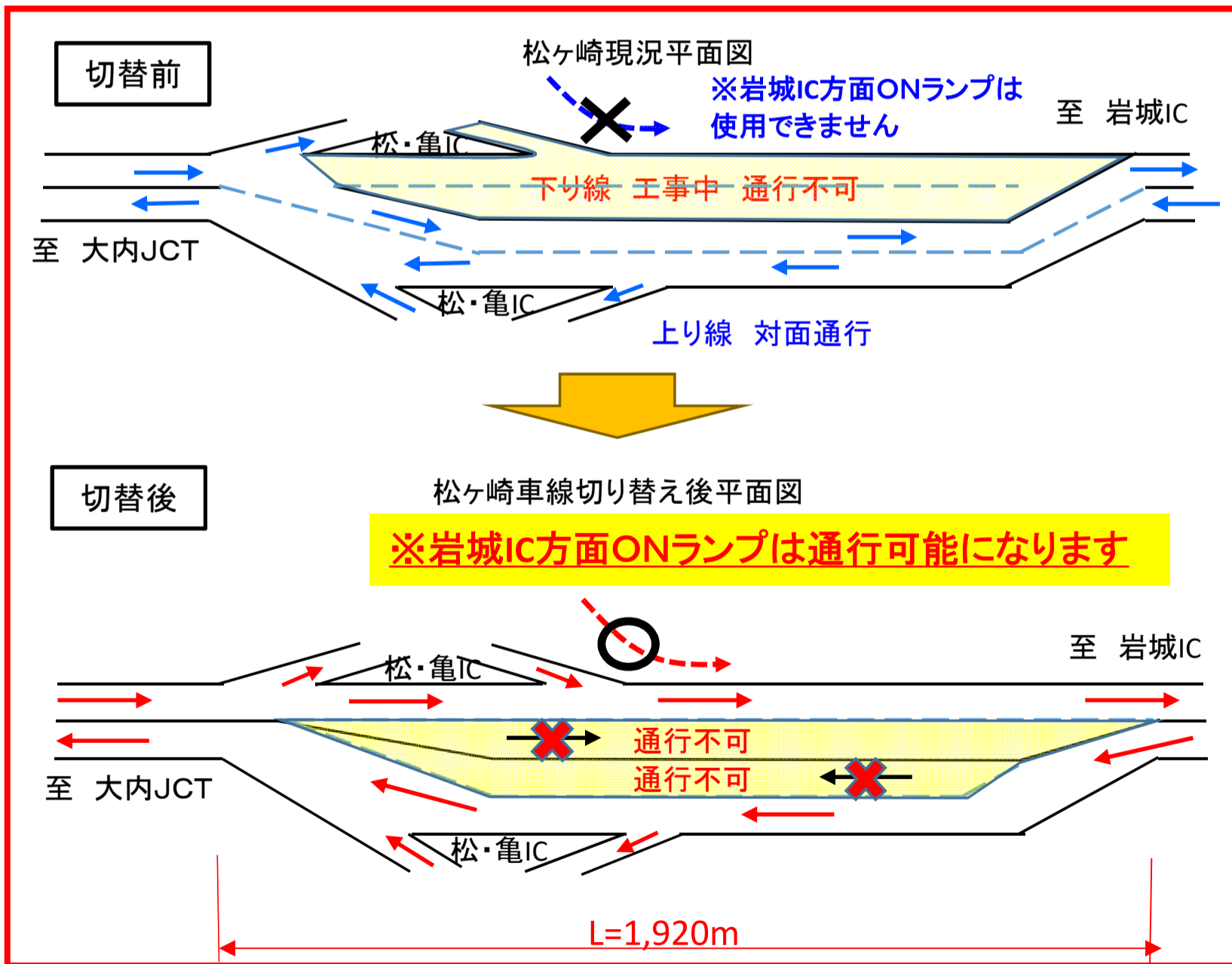
◎車線切り替え前後平面図
