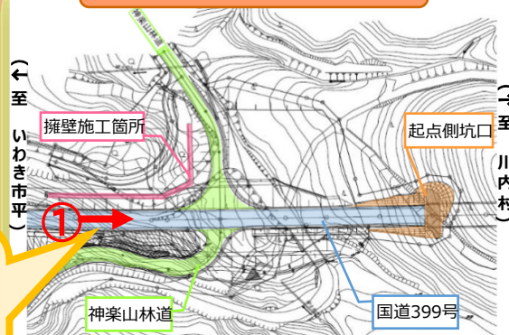
現在、道路になる部分の擁壁をつくっています。
