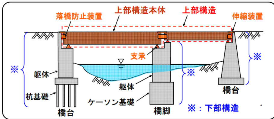
出典)中国地方整備局:橋梁の基礎知識と点検のポイント
