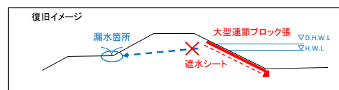
西大塚上流地区河道掘削工事(川西町)
