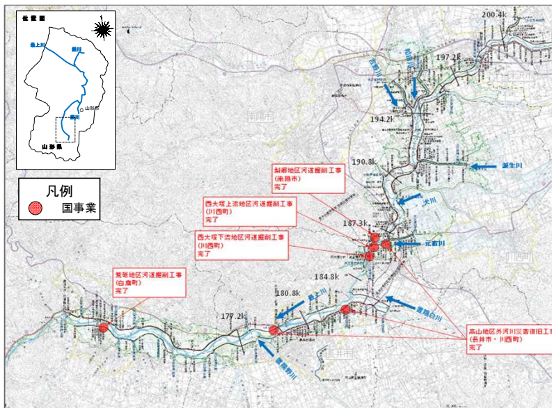
荒砥地区河道掘削工事(白鷹町)
