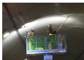
近接目視によるトンネル点検
