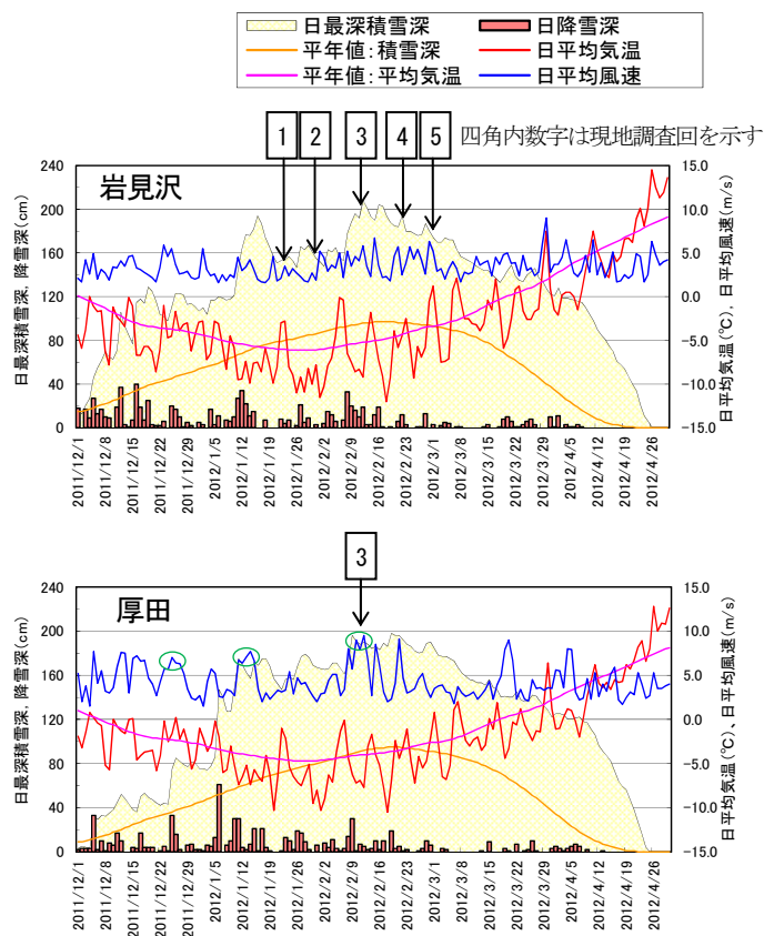
図4 2011年度冬期気象データ (上図岩見沢, 下図厚田)
