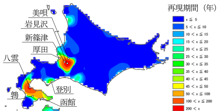
図1 2011年度冬期最大積雪深の再現期間の等値線図 6)
