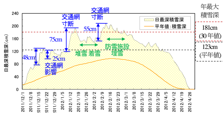
図8 2011年冬期アメダス岩見沢積雪深と道路雪害
