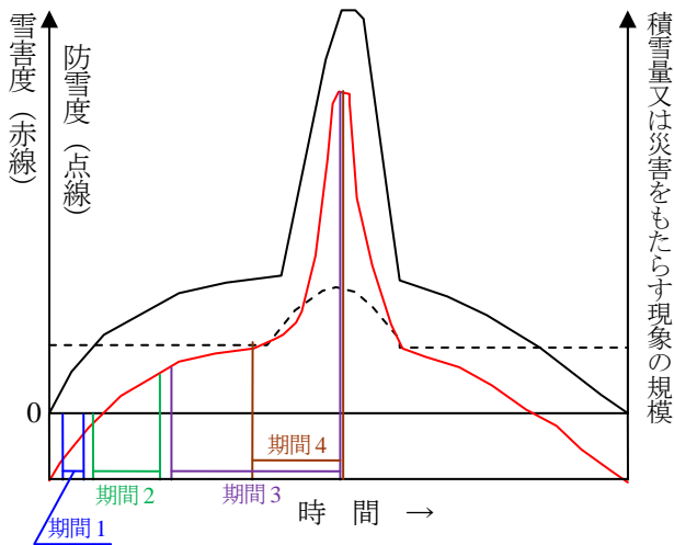
図9 積雪量と防雪度、雪害度との関係 中村 10) を改変 \text{雪害度} = \text{積雪量又は災害をもたらす現象の規模} - \text{防雪度} 期間1から期間4は、表4を参照
