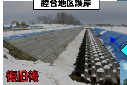
睦合地区護岸
