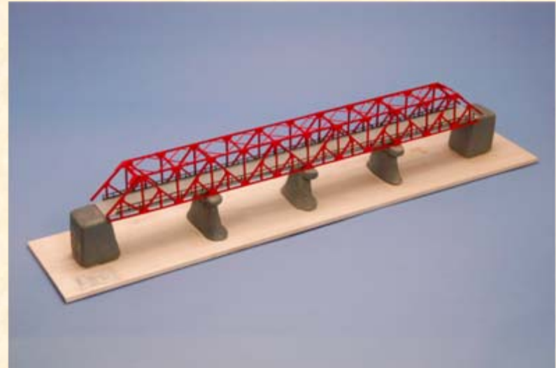
作品名 桜の目橋 学校名 宮城県古川工業高等学校 学 科 土木情報科 作成者 菅原 良太 (3年) 紺野 呼人 (3年) 佐々木 希 (3年) 菅原 秀穂 (3年) 角田 真樹 (3年)
