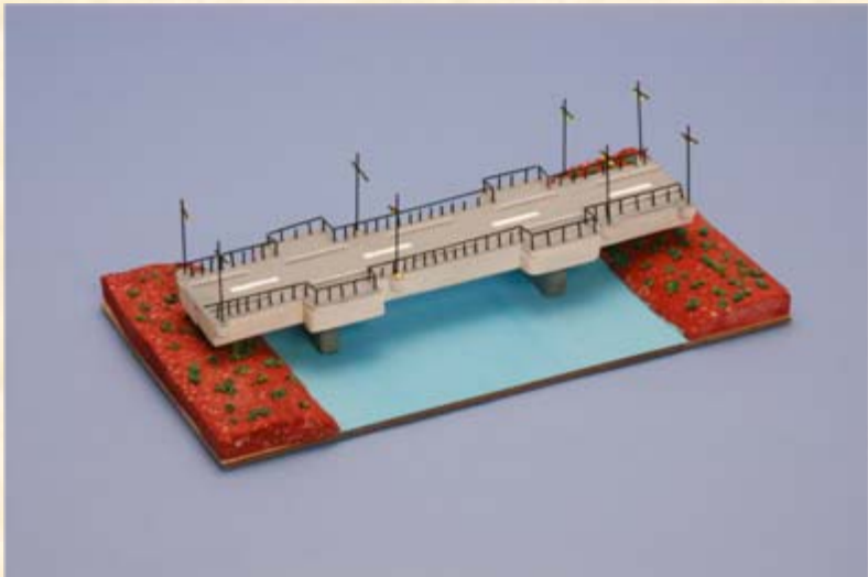
作品名 丸子橋 学校名 秋田県立秋田工業高等学校 学 科 土木科 作成者 田中 茉央 (3年) 佐藤 佑哉 (3年)
