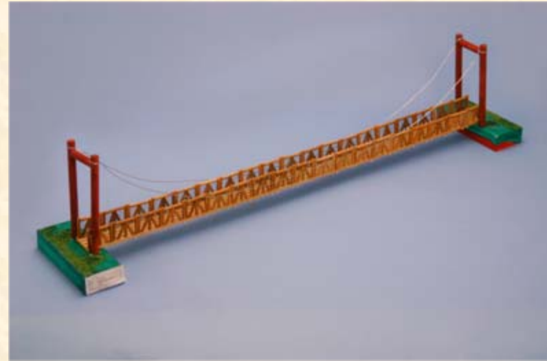
作品名 水天宮吊橋 学校名 青森県立青森工業高等学校 学 科 建築科 作成者 鈴木 諒 (3年) 山崎 拓哉 (3年)
