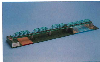
審査員特別賞 | JR 左沢線 最上川橋梁 山形県立寒河江工業高等学校 土木科 落合 亮太 (3年) 佐藤 省吾 (3年) 山田 俊希 (3年) 結城 光 (3年)
