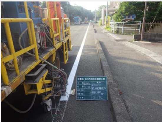
▲施工状況
