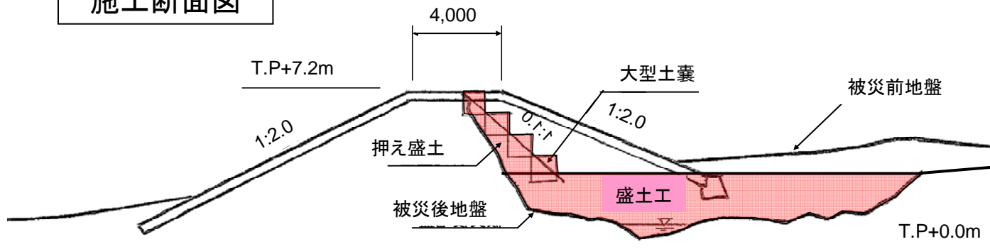
施工断面図
