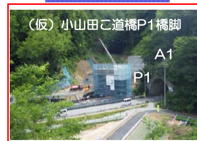
(仮)小山田公道橋P1橋脚では、梁部の型枠組立を行っています。
