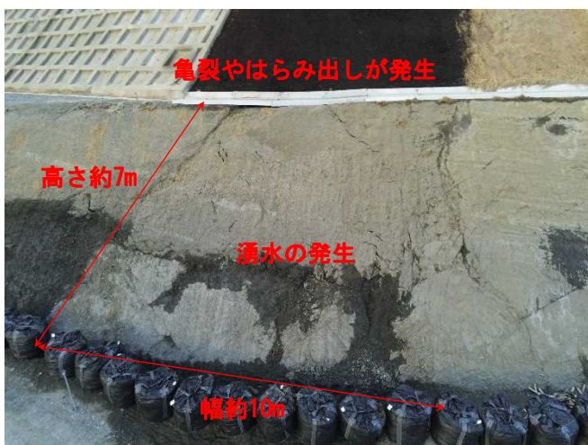
法面変状状況
