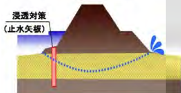
【浸透対策(止水矢板)イメージ】
