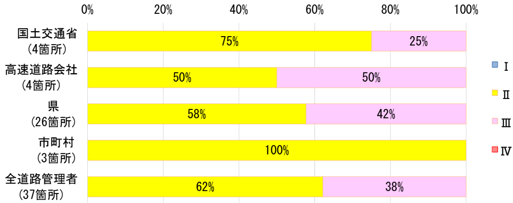
図 3-8 2 巡目 (2019~2022 年度) の判定区分の割合 (トンネル)
