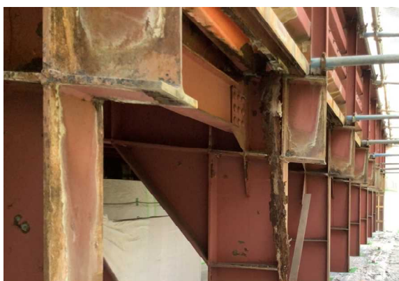
写真 4-20 【損傷】鋼部材の腐食
