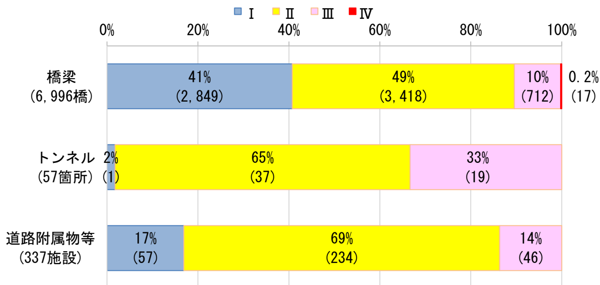
図3-22 2022年度末時点の判定区分の割合（全道路管理者）
