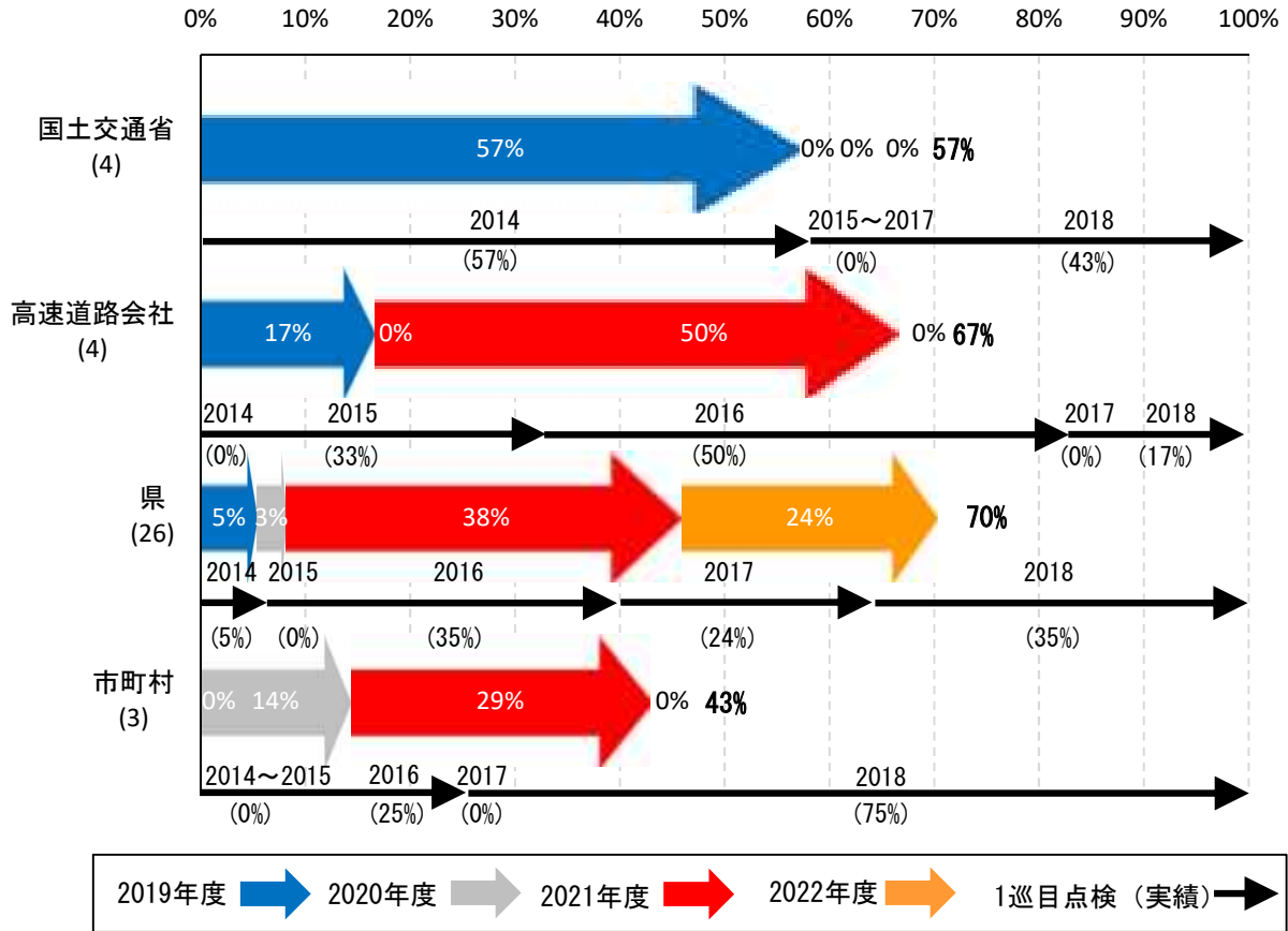
〇2巡目（2019～2022年度）の点検実施率（トンネル）
