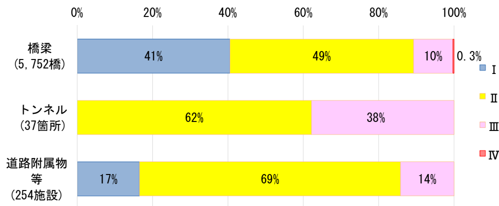
図 3 - 2 2 巡目 (2019~2022 年度) の判定区分の割合 (全道路管理者合計)
