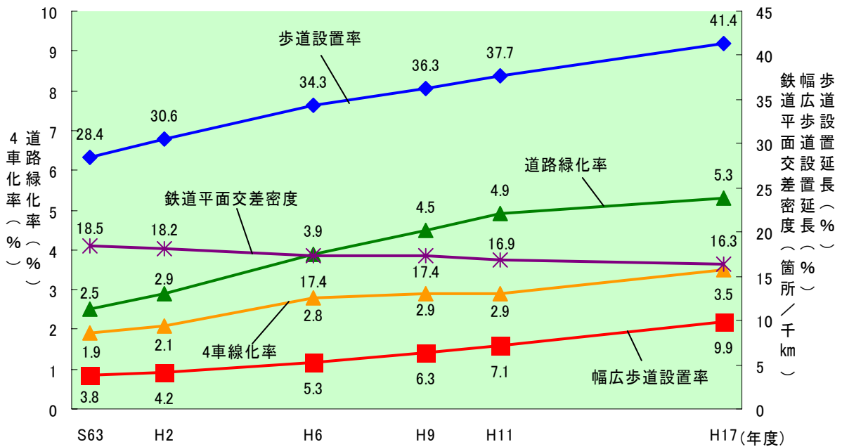
図 一般道路の整備水準の推移(東北管内)
