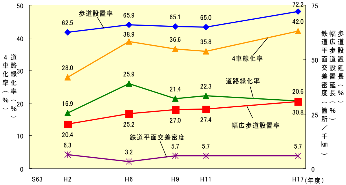
図 一般道路の整備水準の推移(仙台市)
