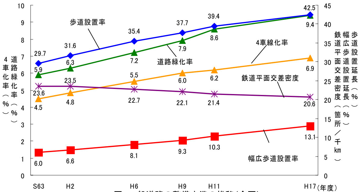
図 一般道路の整備水準の推移(全国)
