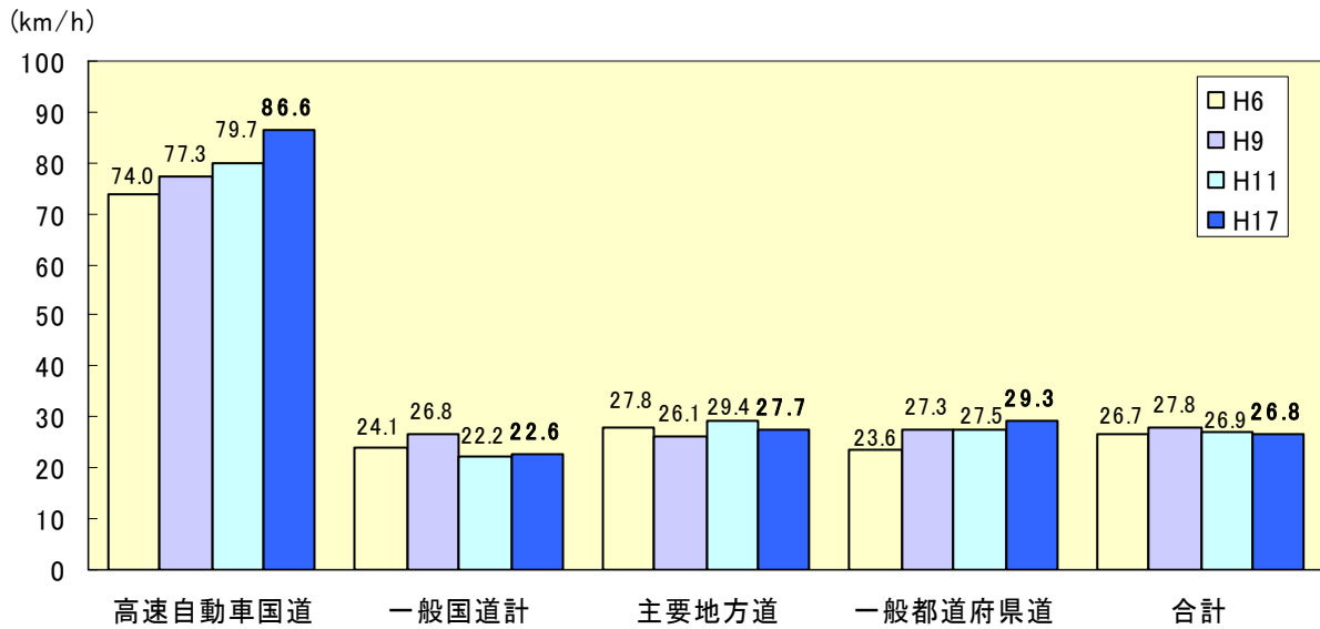
図 道路種別別混雑時旅行速度の推移(平日／仙台市)
