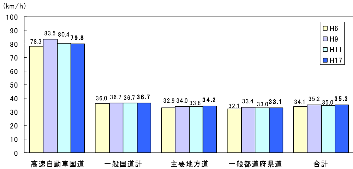
図 道路種別別混雑時旅行速度の推移(平日/全国)
