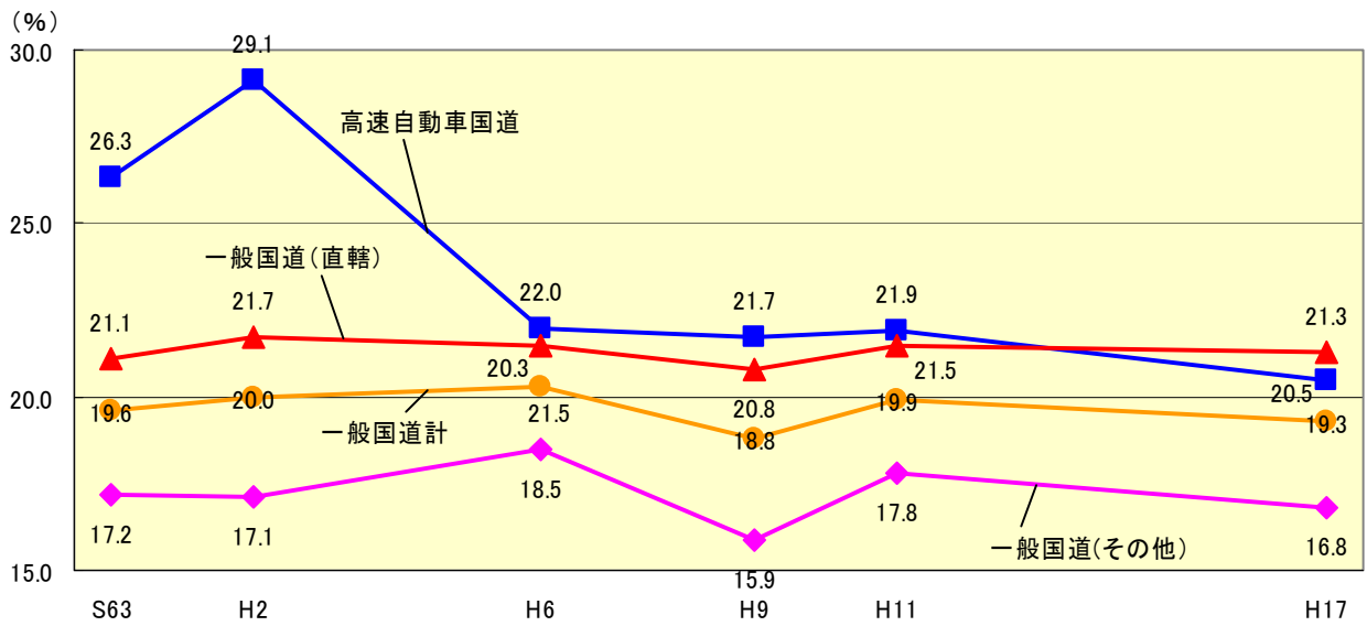
図 道路種別別夜間交通量比の推移(秋田県)
