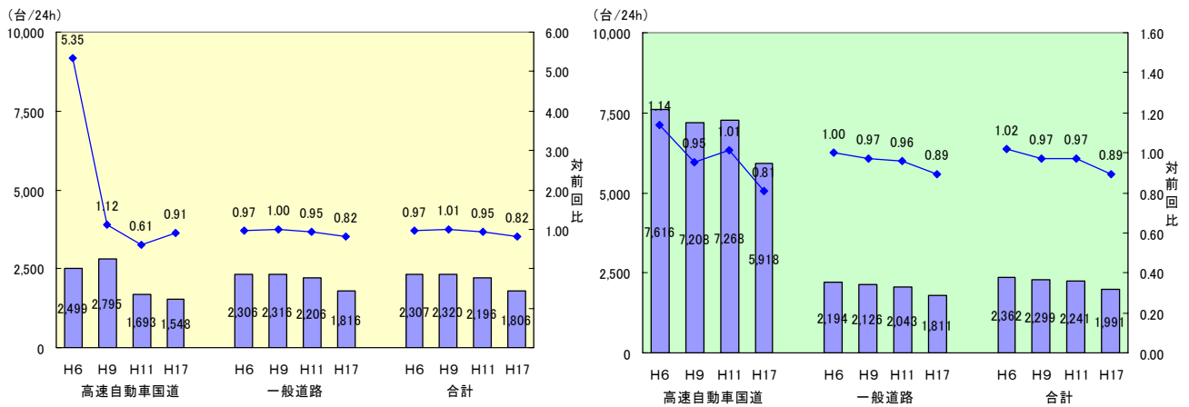
図 車種別平均交通量の推移(貨物車) 左:山形県、右:東北管内計
