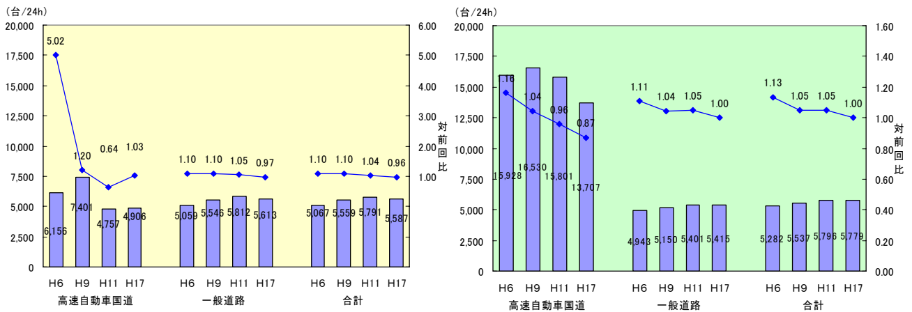
図 車種別平均交通量の推移(全車) 左:山形県、右:東北管内計
