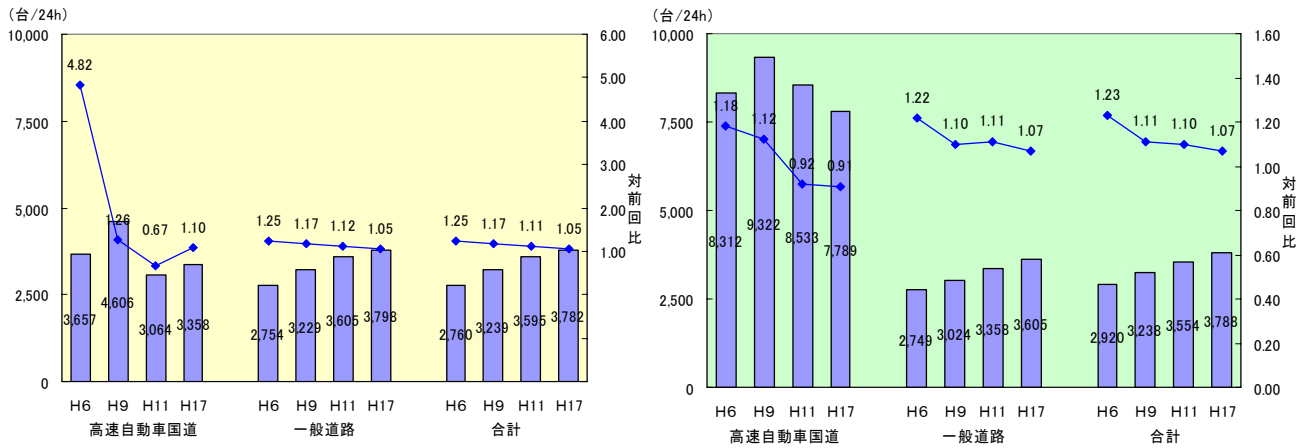
図 車種別平均交通量の推移(乗用車) 左:山形県、右:東北管内計
