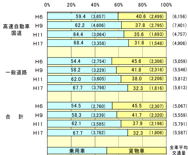
図 平均交通量の車種別構成比の推移(山形県)
