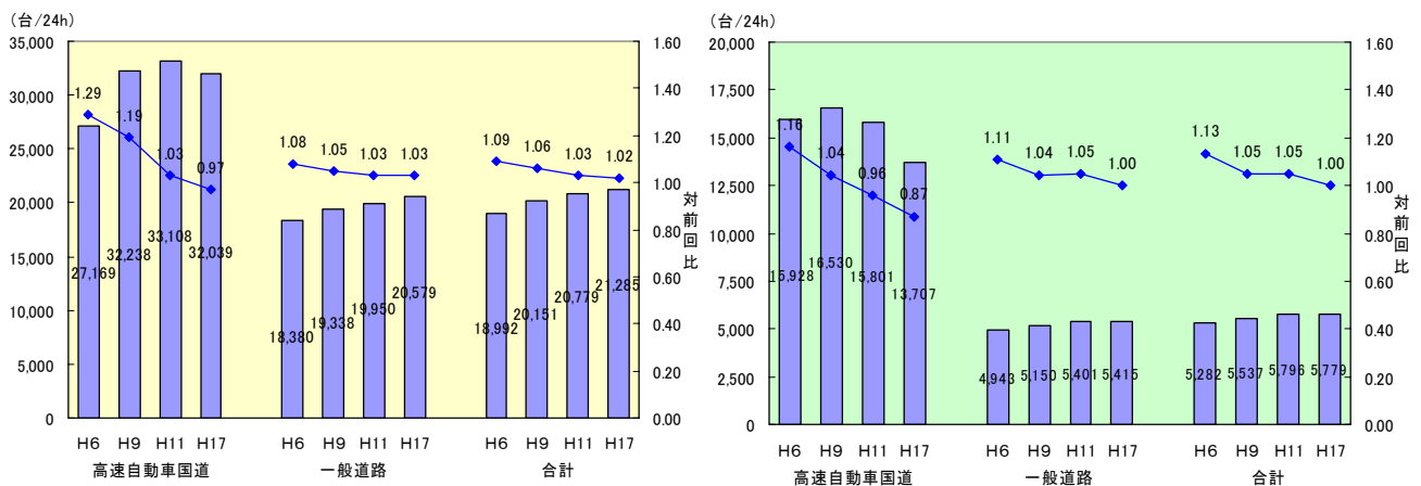
図 車種別平均交通量の推移(全車) 左:仙台市、右:東北管内計
