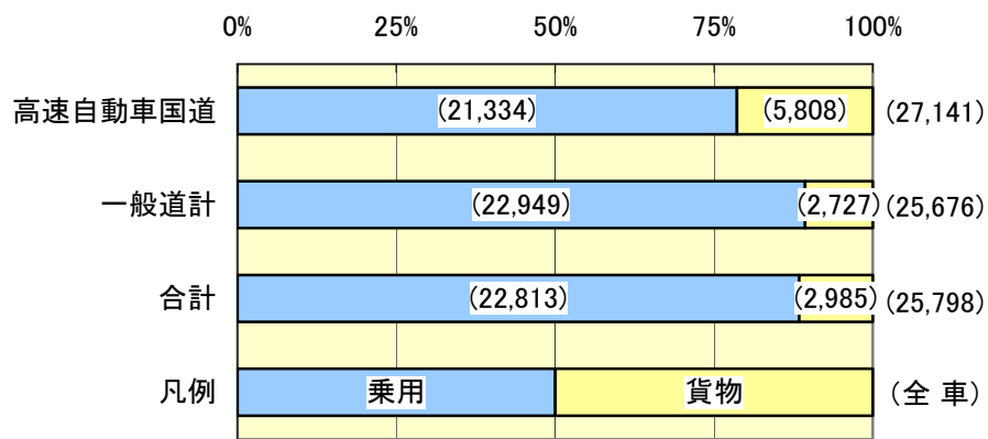
図 平成 17 年度車種別休日平均交通量(仙台市)
