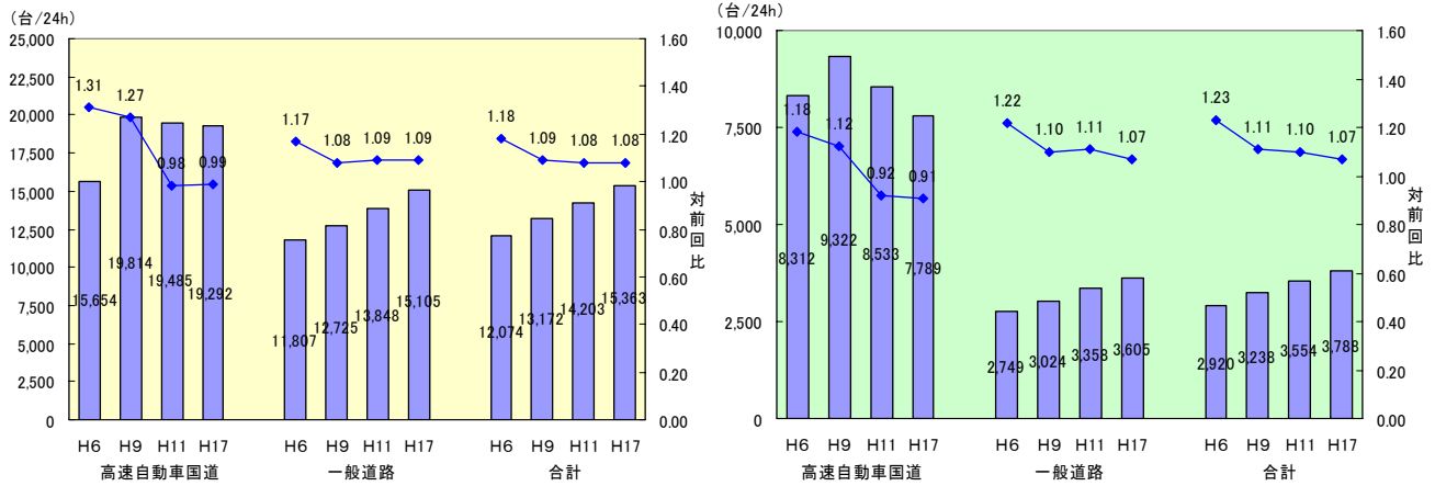
図 車種別平均交通量の推移(乗用車) 左:仙台市、右:東北管内計
