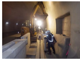
監視員通路立壁設置状況
