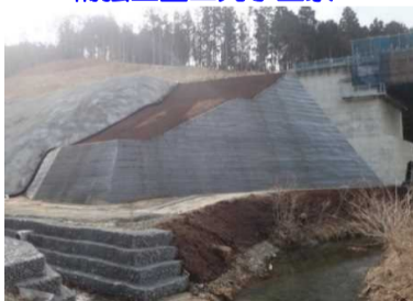
小槌高架橋A1橋台埋戻、補強土壁工完了全景
