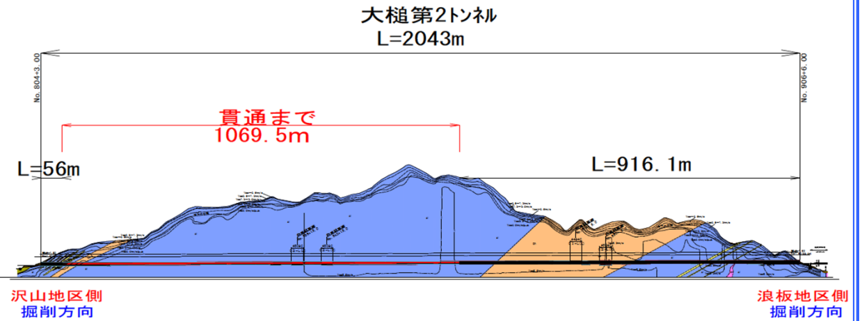
【図】大槌第2トンネルの進捗状況 (掘削延長:H27. 5月20日時点)
