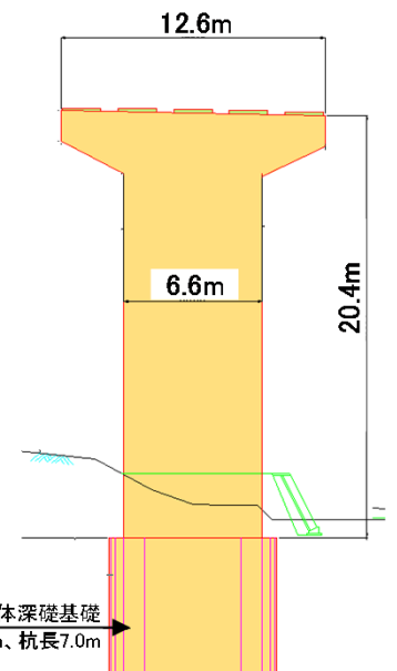
【浪板高架橋 P1橋脚正面図】
