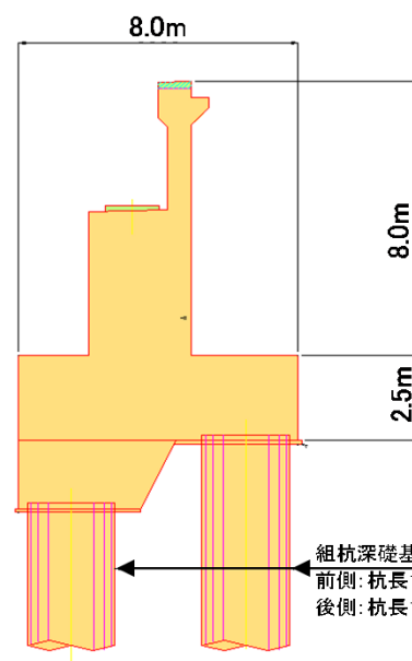
【浪板高架橋 A2橋台断面図】
