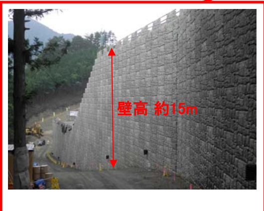
補強土擁壁の施工状況
