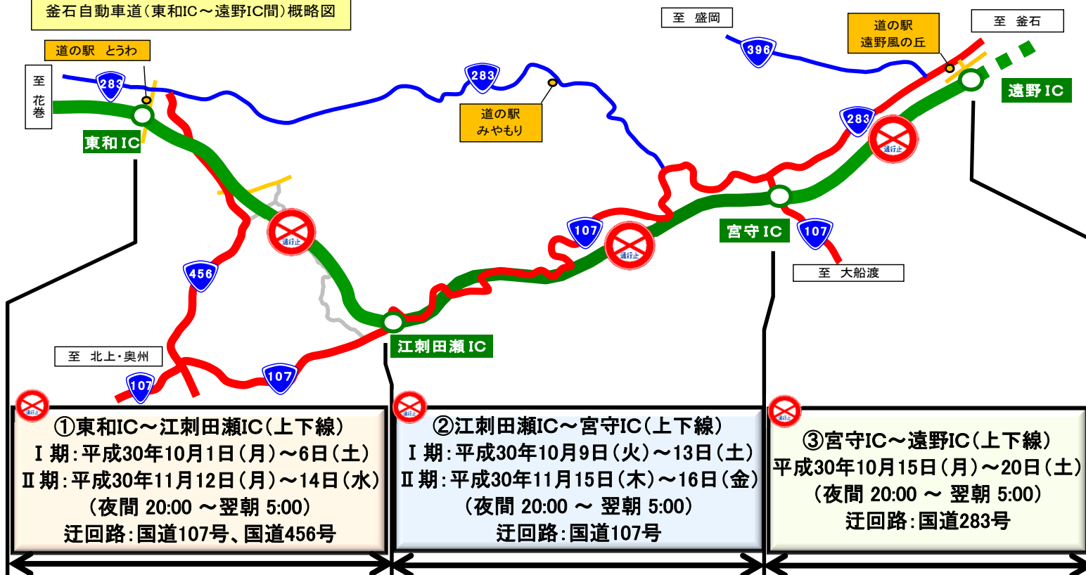
釜石自動車道(東和IC～遠野IC間)概略図
