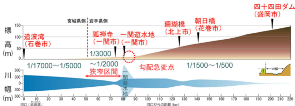
北上川の河床勾配と川幅
