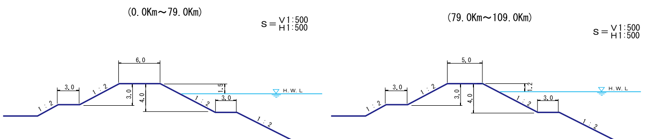
阿武隈川上流堤防標準断面図
