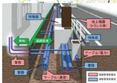
電線共同溝イメージ
