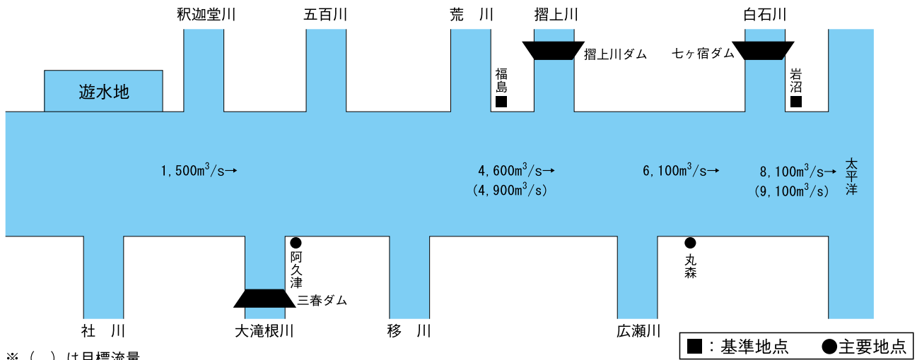
阿武隈川における河道配分流量
