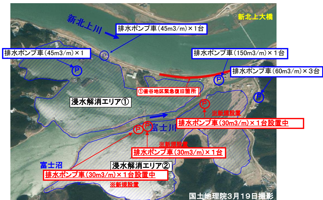
石巻市針岡 4月5日 排水ポンプ車による排水位置状況(30m 3 /m 3台追加配備)
