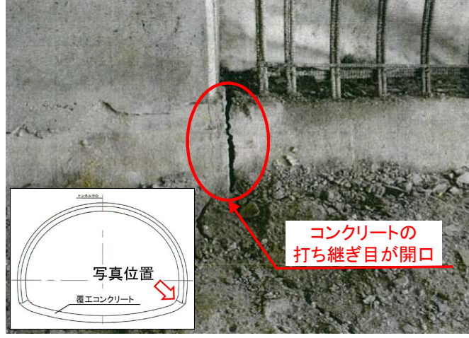
【(仮称)前波トンネル終点側(酒田側)覆工コンクリート状況】
