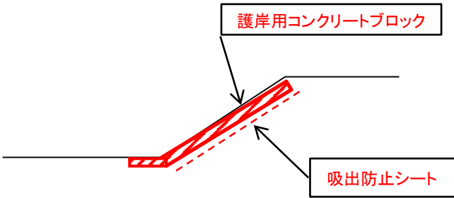
標準断面のイメージ
