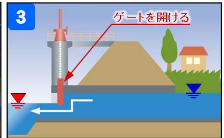
河川の水位が下がれば、ゲートを開けて溜まった水を排水
