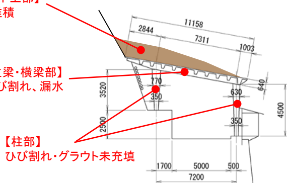
▲シェッド標準断面図
