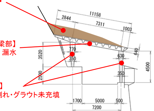
▲シェッド標準断面図
