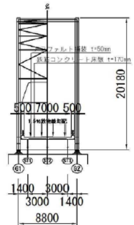
▲標準断面図
